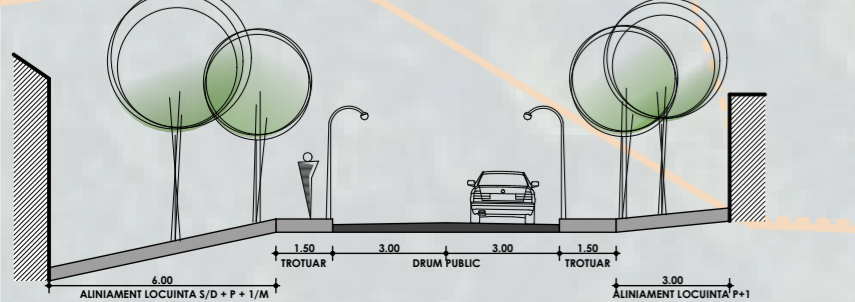
PROFIL STRADA A TRONSON 1
