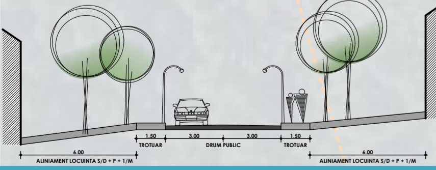
PROFIL STRADA A TRONSON 1
